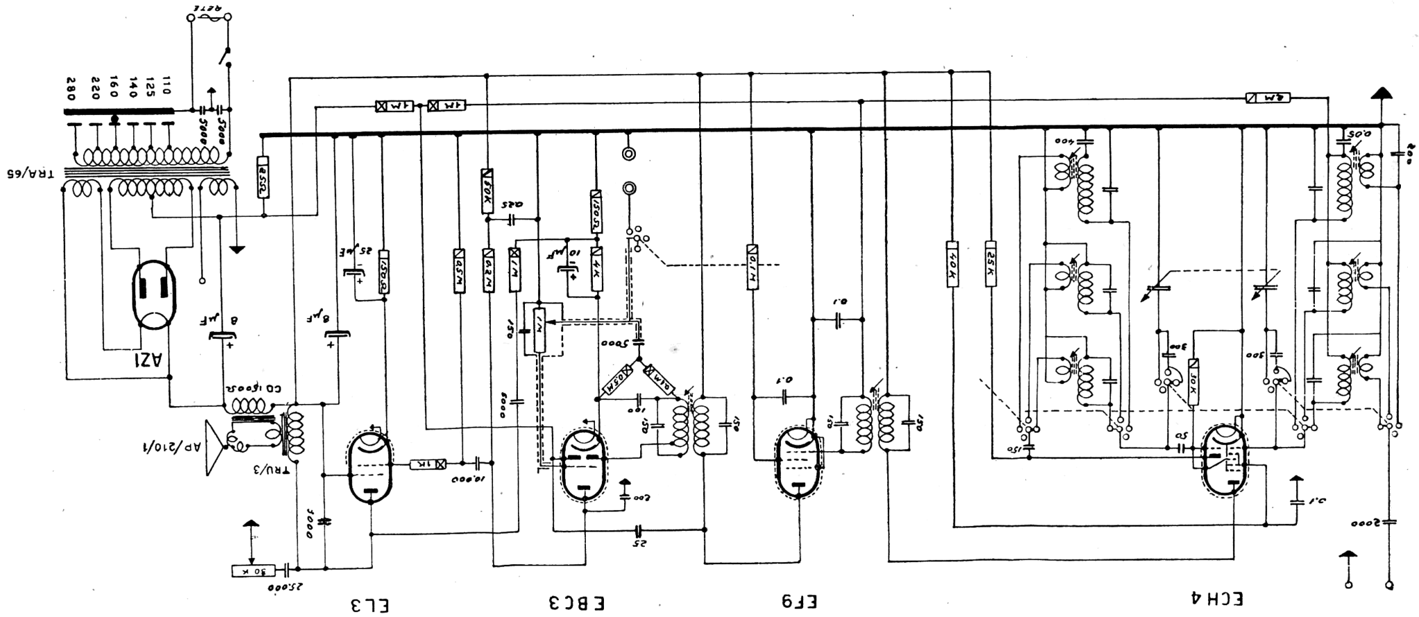
BERTONCINI RADIO - Mod. LEILA 1. Una gamma onde medie, due gamme onde corte. Reazione negativa al catodo della EBC3. Media frequenza: 468 kc. Sensibilità media: 20 \mu V. Bobina campo: 1500 ohm. Potenza d'uscita: 3 watt.
